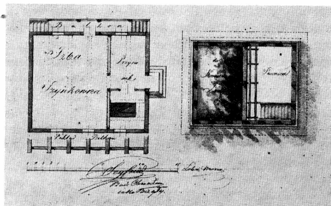
Ryc. 12. Rzut kamieniczki w Szczuczynie — „Domu Szynekowego”, fot. ze zbiorów PIS w Warszawie
